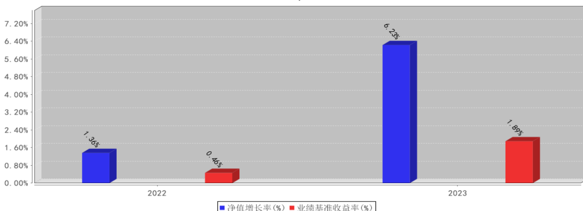
方正富邦稳丰一年定开债券发起基金每年净值增长率与同期业绩比较基准收益率的对比图（2023年12月31日）
